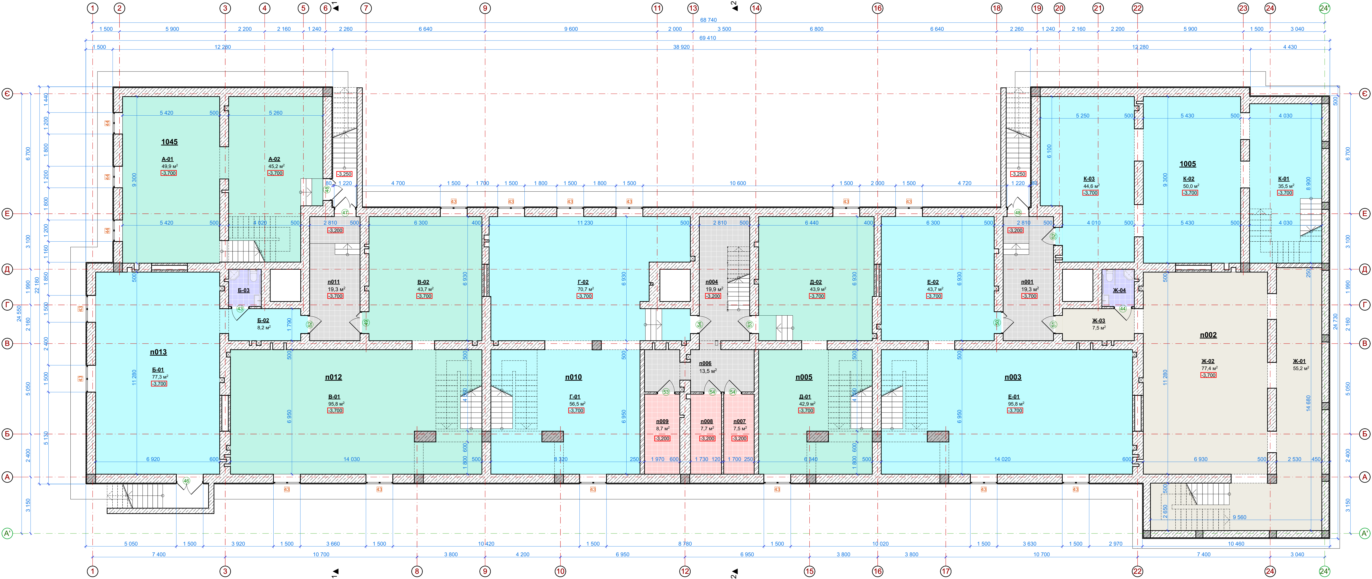
План підвалу /м 1:100/
