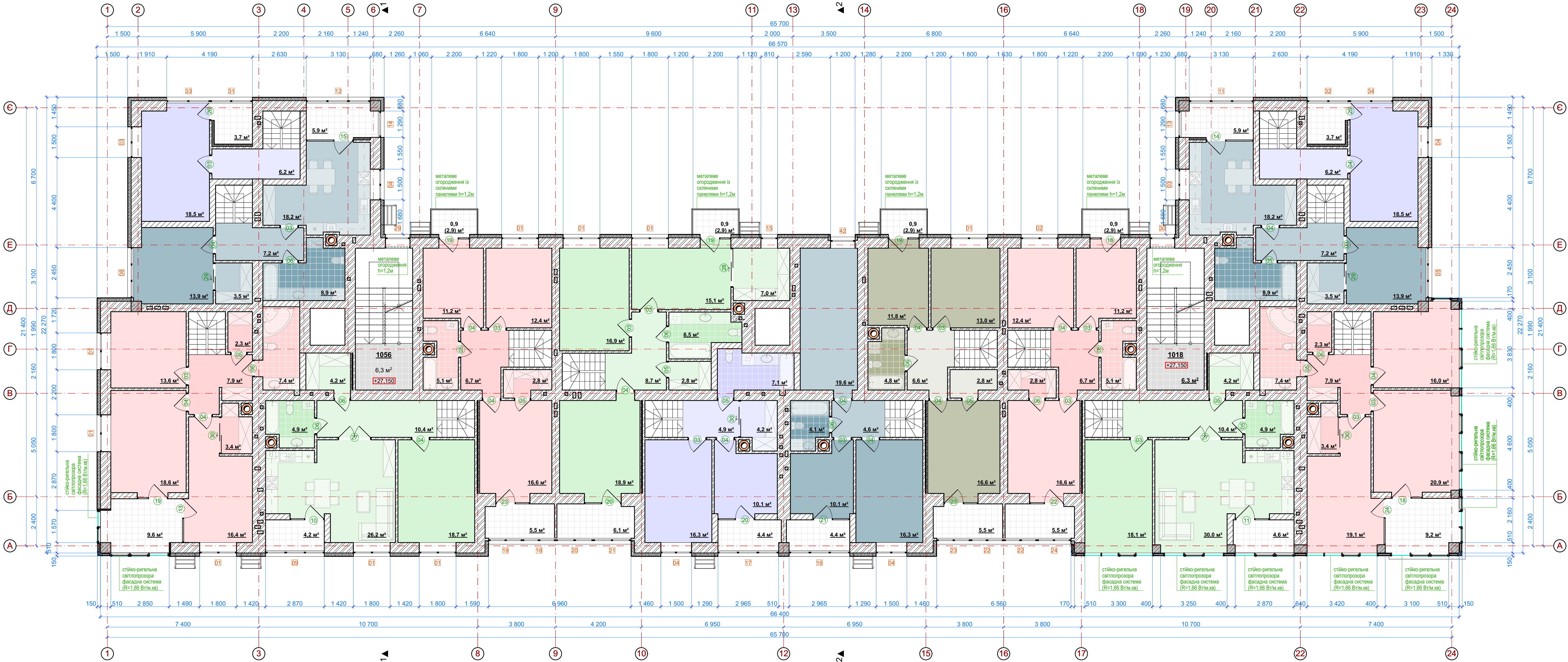
План 10-го поверху (II-ий рівень дворівневих квартир) /м 1:100/
