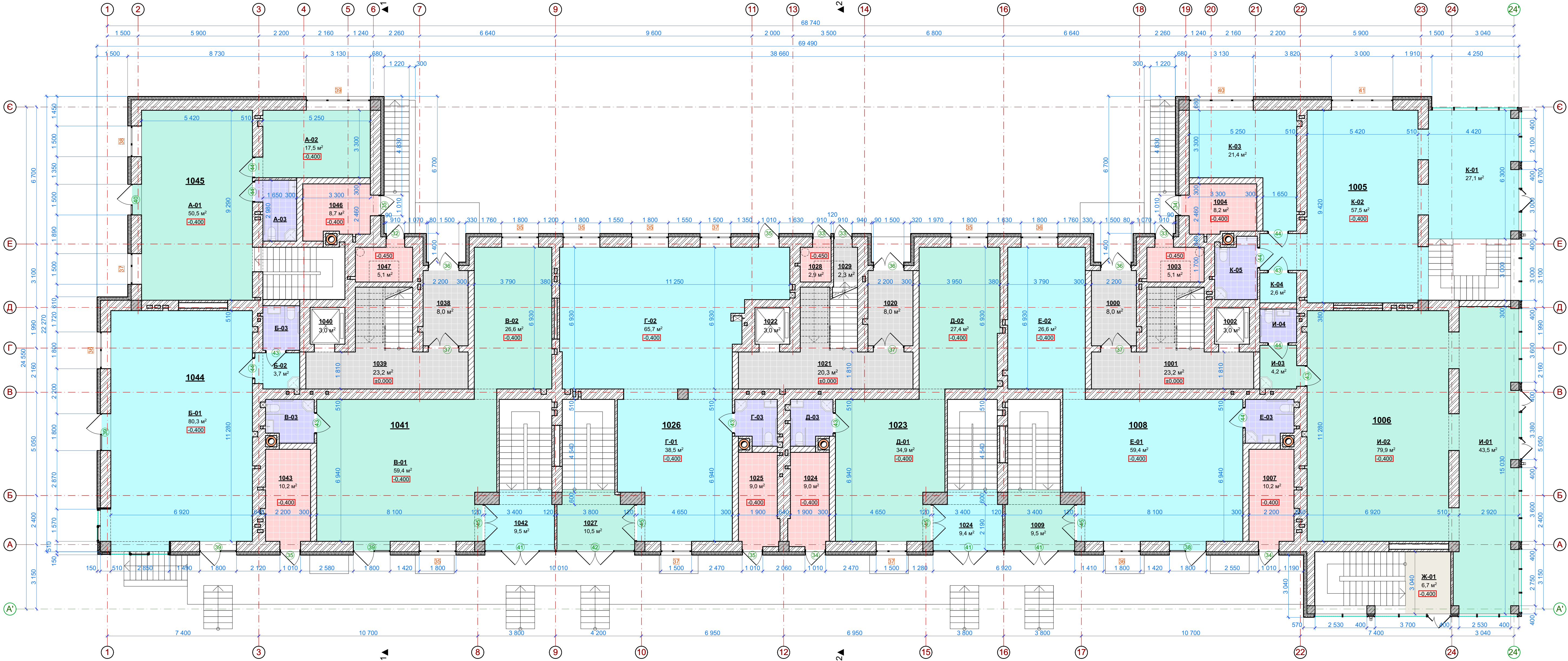
План 1-го поверху /м 1:100/
