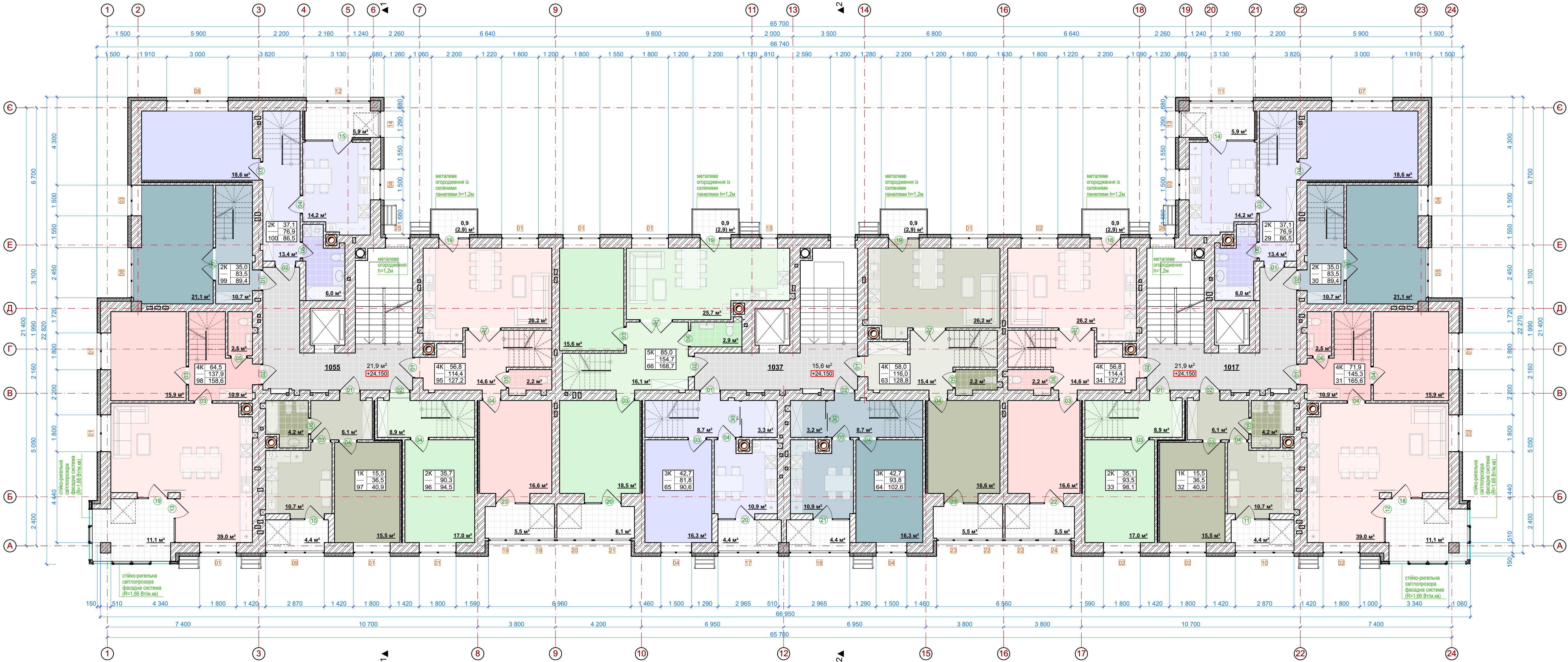
План 9-го поверху (І-ий рівень дворівневих квартир) /м 1:100/
