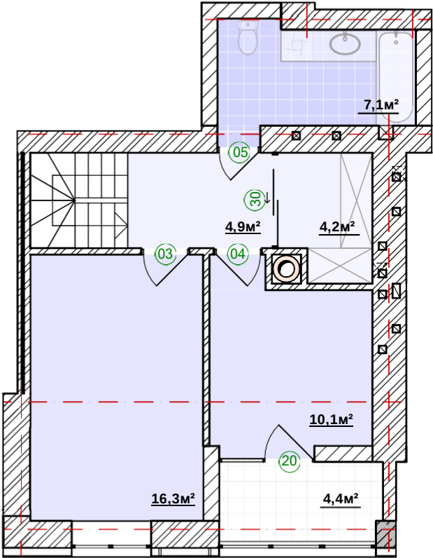
План2-горівняквартири(вмежах10-гоповерху)
