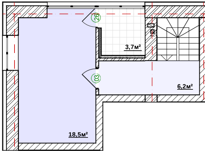
План2-горівняквартири(вмежах10-гоповерху)
